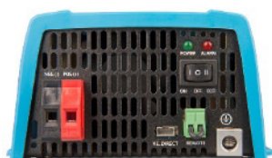
Wechselrichter 12/375 VE.Direct
