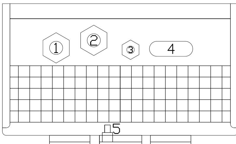
Figura 1. Vista dal basso dell'armadio in cui sono visibili gli ingressi dei cavi: modelli a due uscite
