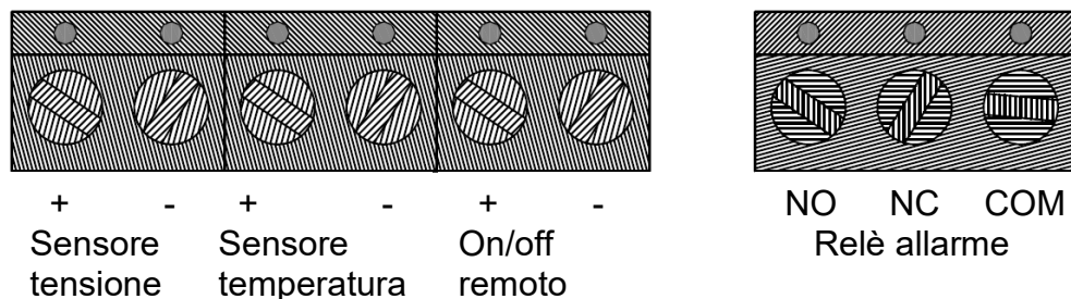
Figura 5: Blocco di collegamento
