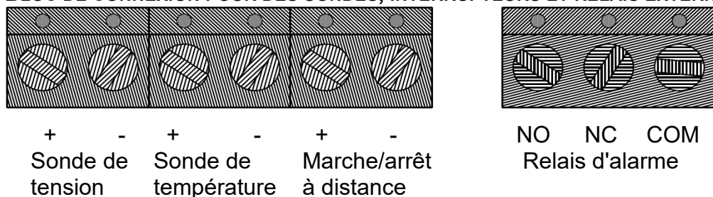
Figure 5. Bloc de connexion
