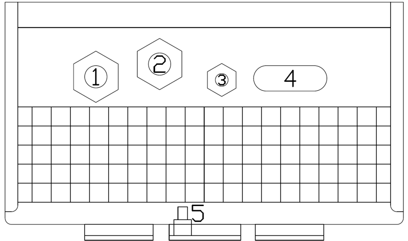
Abbildung 1. Gehäuse von unten mit Sicht auf die Kabeleinführungen: Modelle mit zwei Ausgängen
