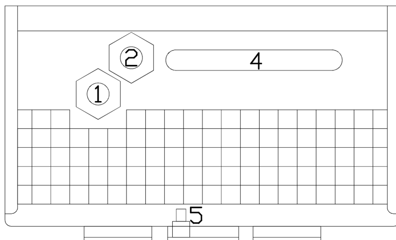
Figura 2. Vista dal basso dell'armadio in cui sono visibili gli ingressi dei cavi: modelli a tre uscite
