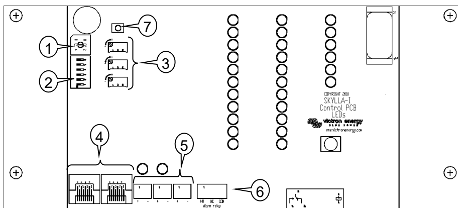
Figura 7. Comandi interni e collegamenti
