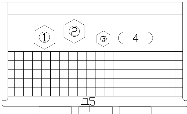
Figure 1. Vue inférieure de l'armoire montrant les entrées de câbles : modèles à deux sorties
